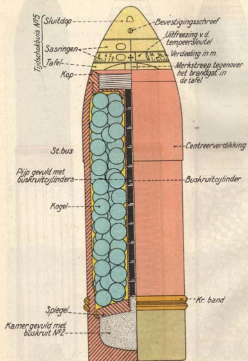
Fig. 41. ( \frac{1}{2} ). Granaatkartets van 7 veld. (In schokstelling)
