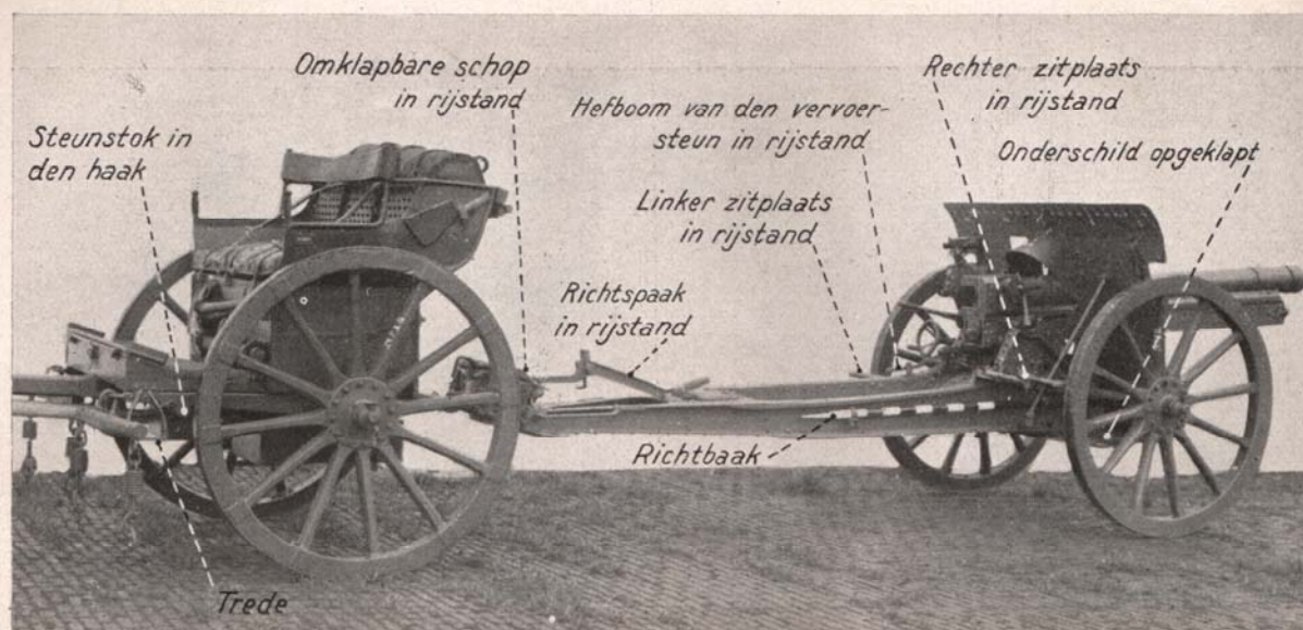
Fig. 2. Vuurmond, opgelegd.
