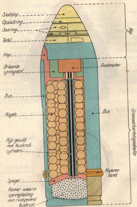
Fig. 43. ( \pm 1/2 ). Brisantgranaatkartets.
