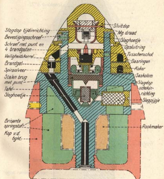
Fig. 44. ( \frac{1}{1} ). Tijdschokbuis No. 12, met kop van de bgkt.
