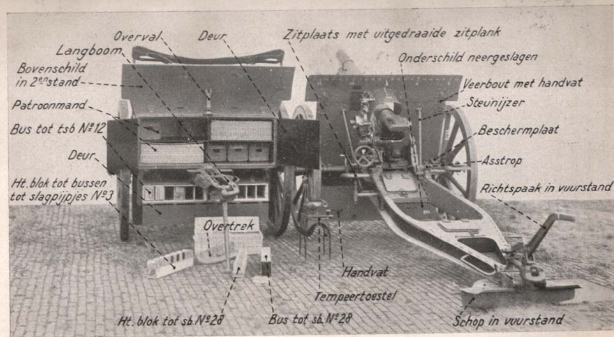
Fig. 3. Stuk in vuurstelling.
