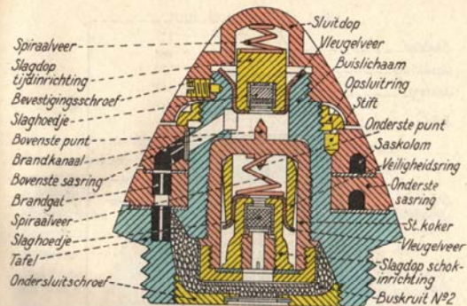
Fig. 42. ( 1/1 ). Tijdschokbuis No. 5.
